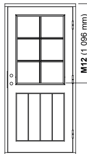
Glashöjd 12 Spröjs 2:1
