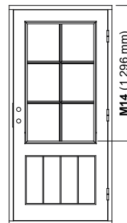
Glashöjd 14 Spröjs 2:1
