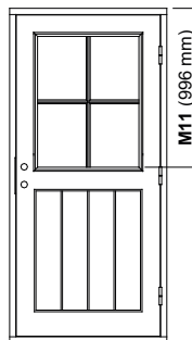
Glashöjd 11 Spröjs 1:1
