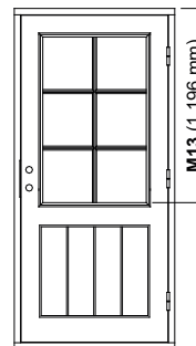
Glashöjd 13 Spröjs 2:1
